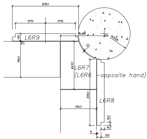
DETAIL D1
